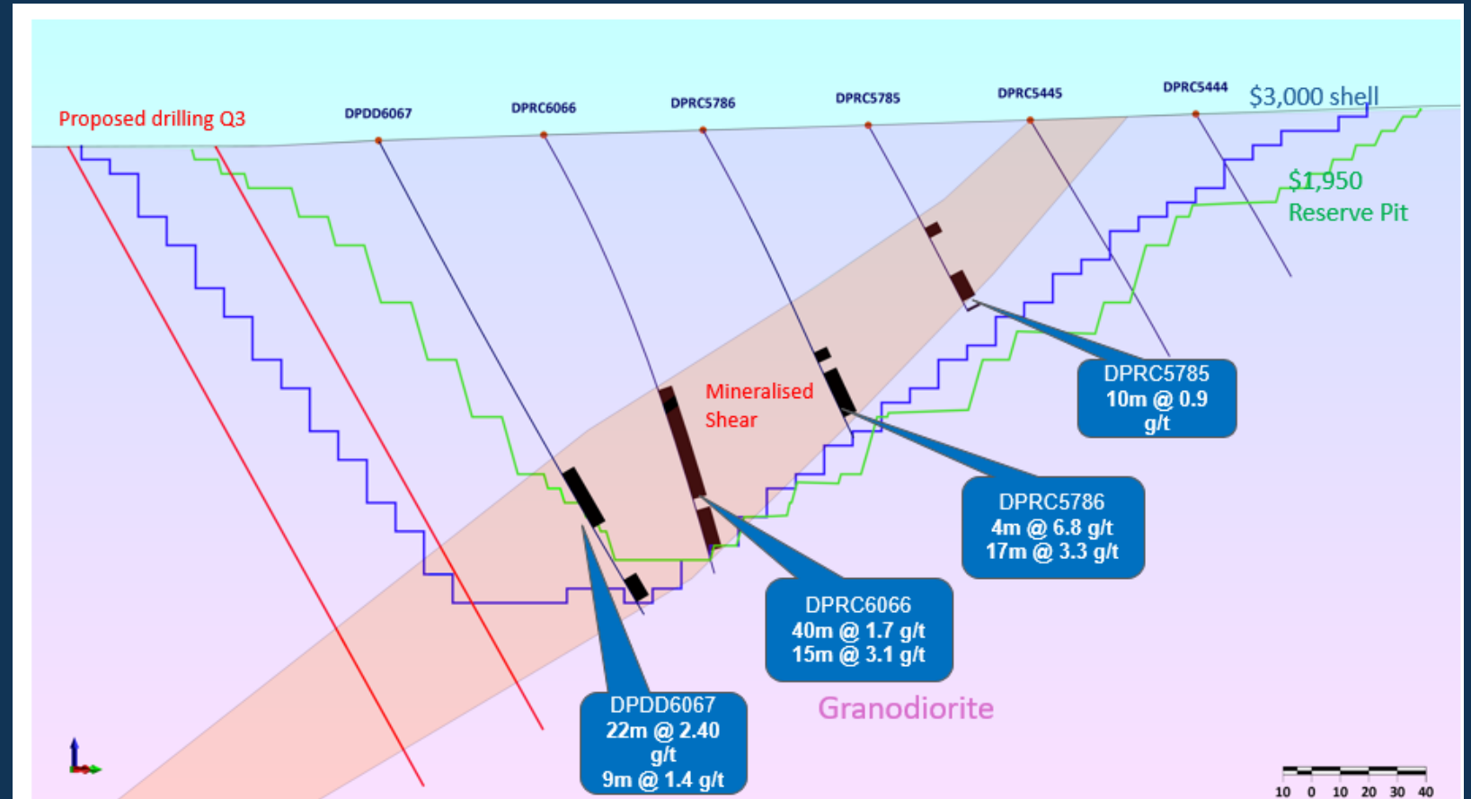
Kilosegui Cross Section
